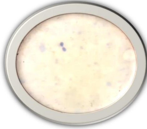
شكل (4) : طبعة من الكبد مصبوغة بصبغة الكيمزا بعد حقن اللشمانيا الحشوية المضعفة المعرضة لليزر اندياك في 500 نبضة بنسبة قتل %89.8.
